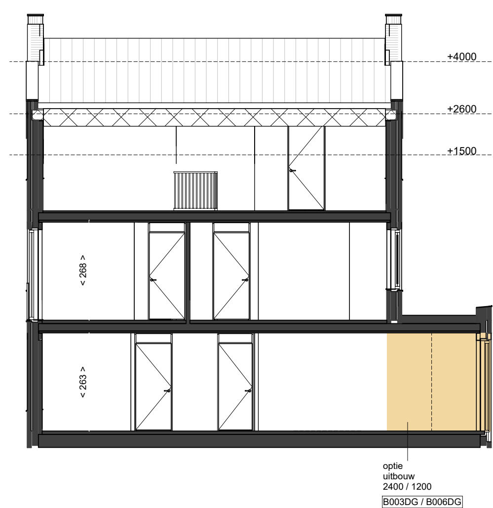
DOORSNEDE
