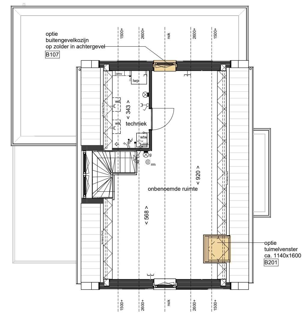
2e VERDIEPING
