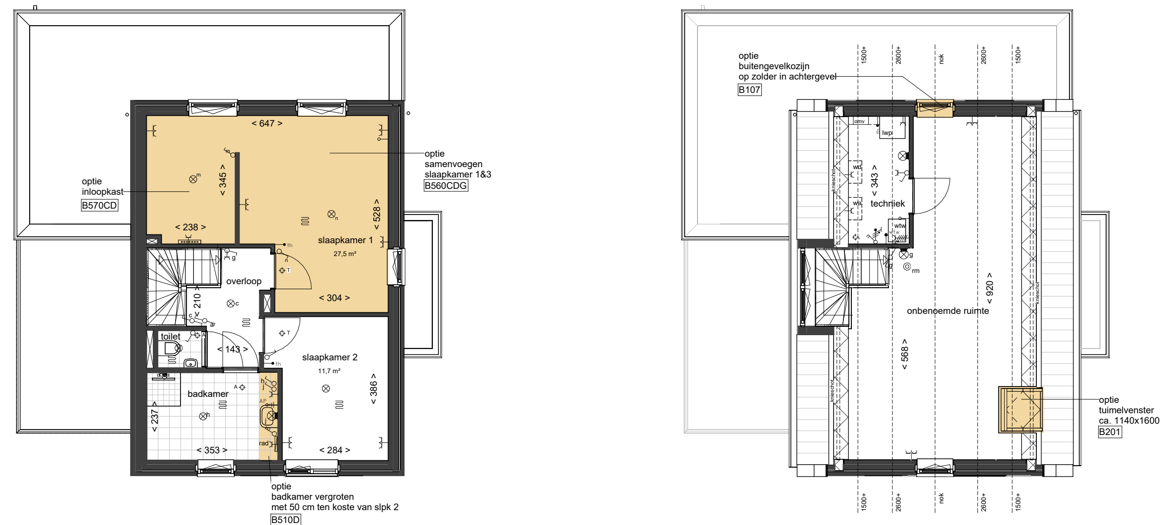
1e VERDIEPING
