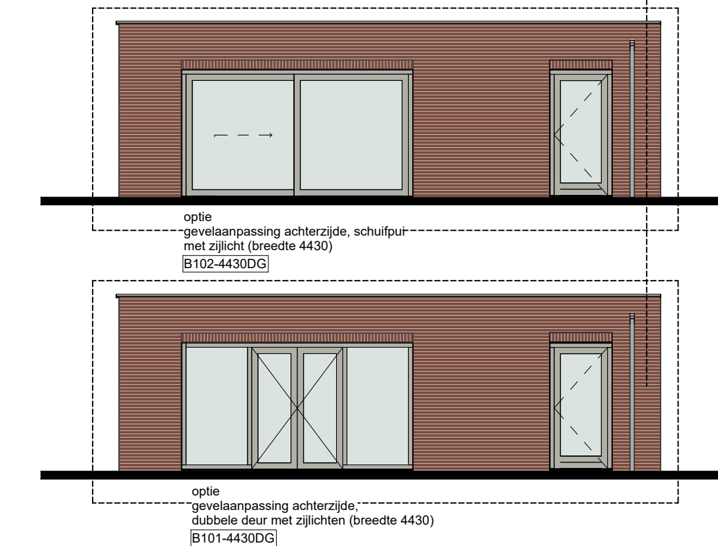
ACHTERGEVEL
